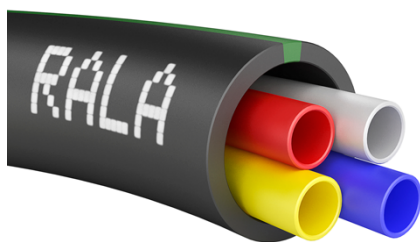
Exempel på 4x12 mm mikrorör i 40/32 mm optorör.
